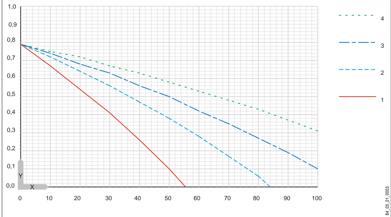
График КПД
