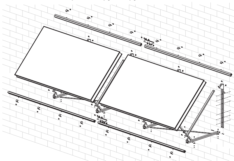
Настенный монтаж рядом друг с другом
