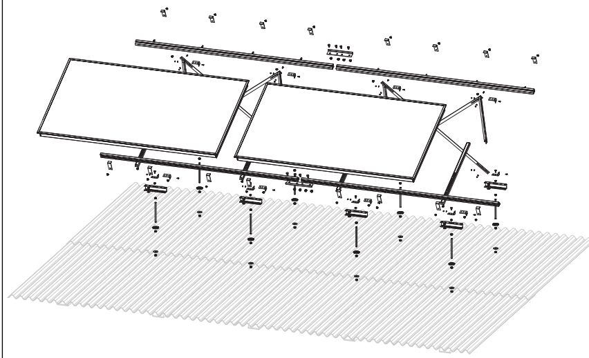
Монтаж на волнистую кровлю рядом друг с другом на основании
