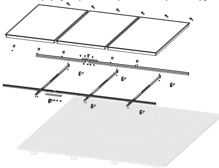
Монтаж на шиферную кровлю вертикально, рядом друг с другом
